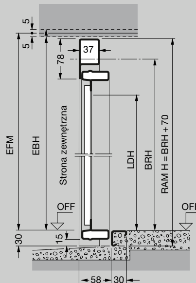
Przekrój pionowy Brama z progiem
