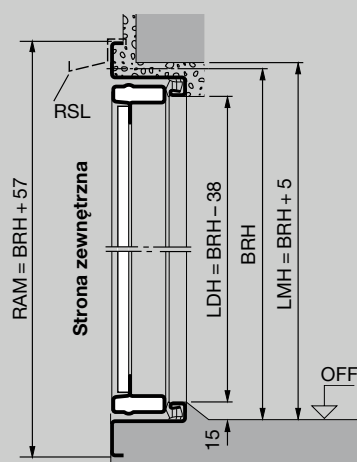
Przekrój pionowy Drzwi z progiem
