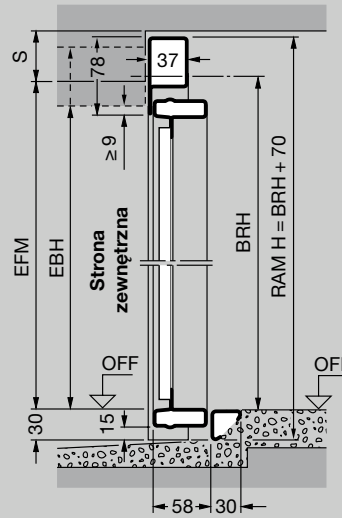
Przekrój pionowy Brama z progiem
