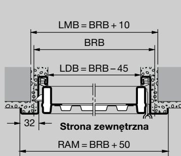
Przekrój poziomy
