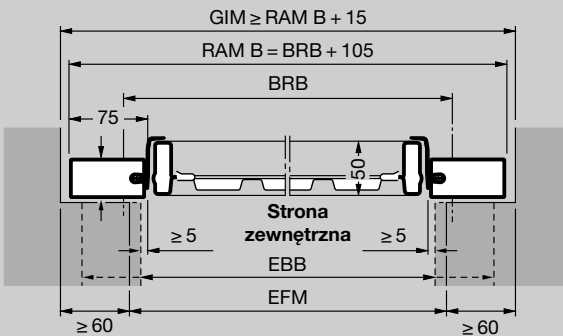
Przekrój poziomy Montaż za otworem
