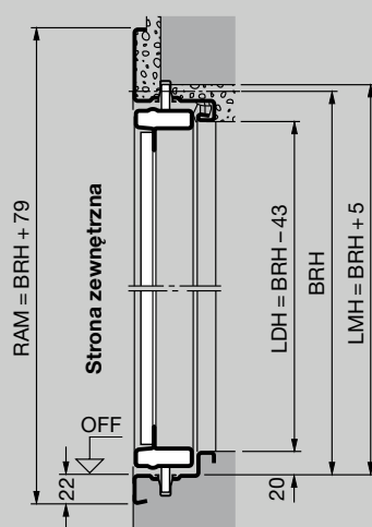
Przekrój pionowy Drzwi z progiem
